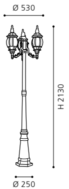
floor luminaire; cast aluminium, black-green / glass, clear Stehleuchte; Aluguss, schwarz-grün / Glas, klar lampadaire; aluminium moulé, noir-vert / verre, clair
