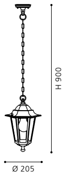
pendant luminaire; cast aluminium, black / glass, clear Hängeleuchte; Aluguss, schwarz / Glas, klar luminaire suspension; aluminium moulé, noir / verre, clair
