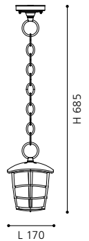
pendant luminaire; cast aluminium, black / plastic, clear Hängeleuchte; Aluguss, schwarz / Kunststoff, klar luminaire suspension; aluminium moulé, noir / plastique, clair
