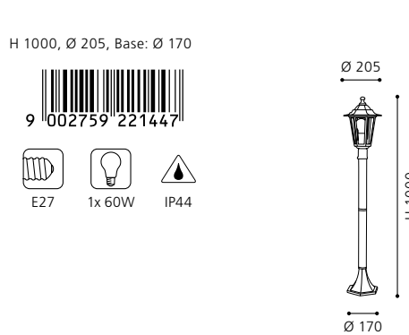
floor luminaire; cast aluminium, black / glass, clear Stehleuchte; Aluguss, schwarz / Glas, klar lampadaire; aluminium moulé, noir / verre, clair
