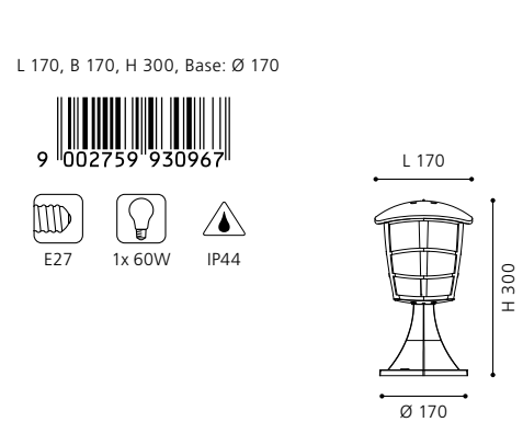
pedestal luminaire; cast aluminium, white / plastic, clear Sockelleuchte; Aluguss, weiss / Kunststoff, klar borne; aluminium moulé, blanc / plastique, clair
