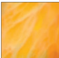
Calcite (CALC)
